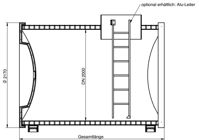
Schnitt A-A
