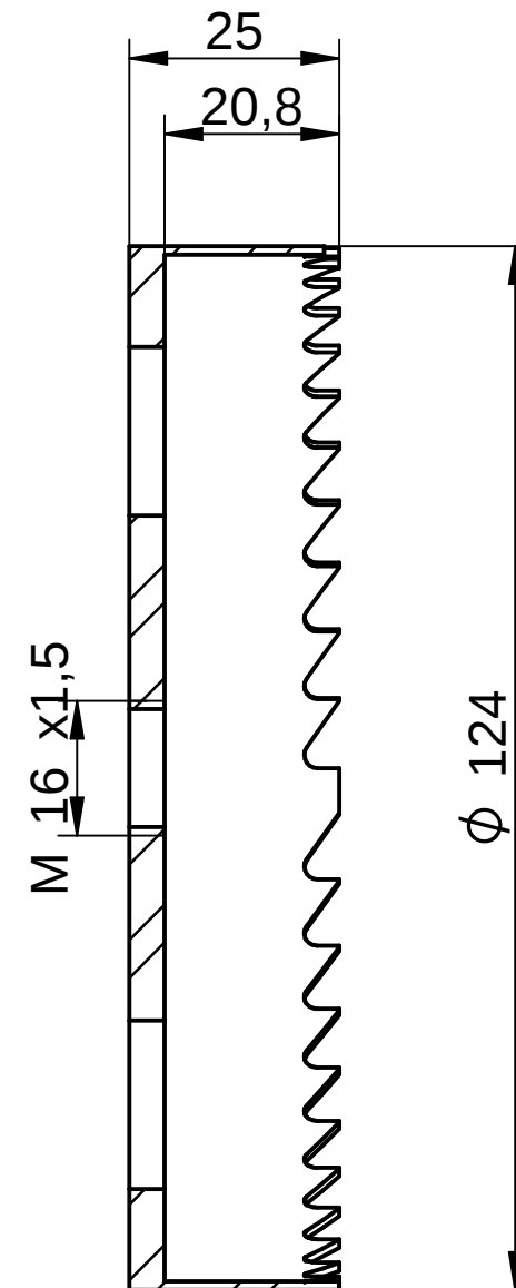
Schnitt A-A
