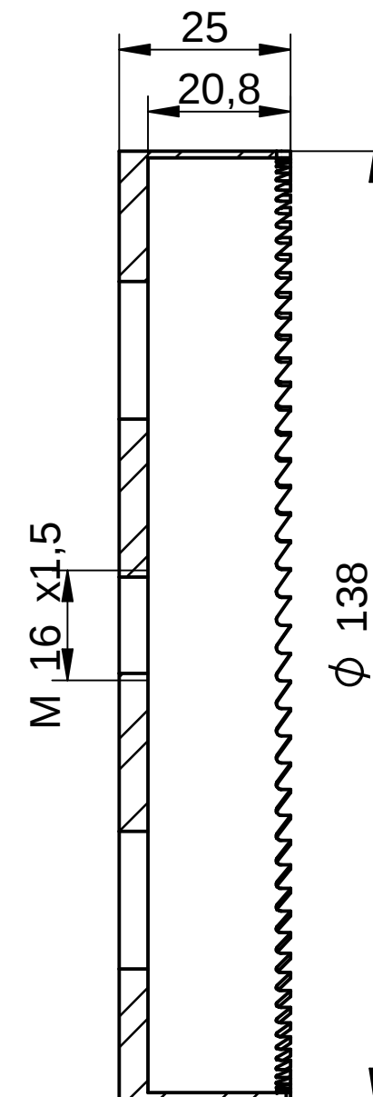
Schnitt A-A
