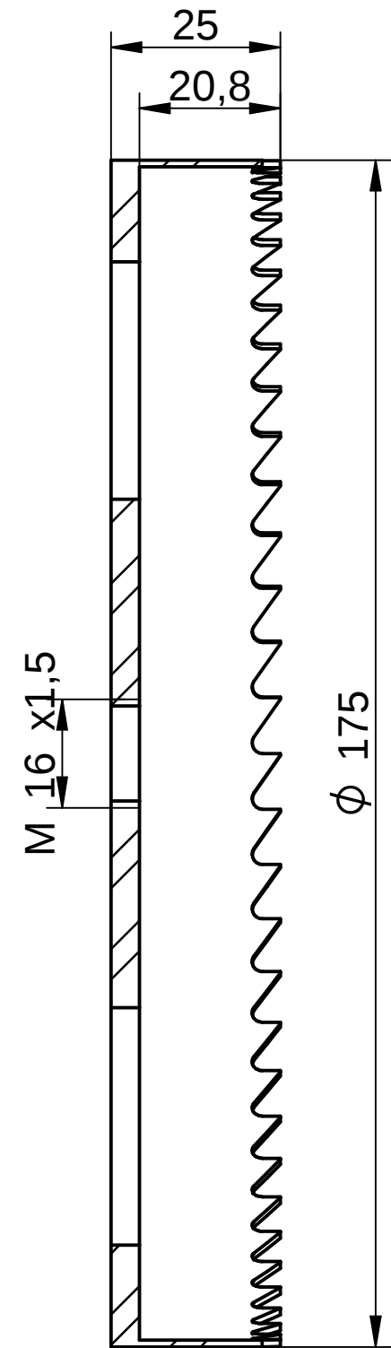
Schnitt A-A
