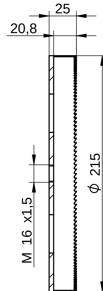
Schnitt A-A
