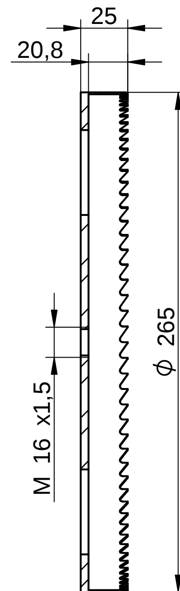
Schnitt A-A
