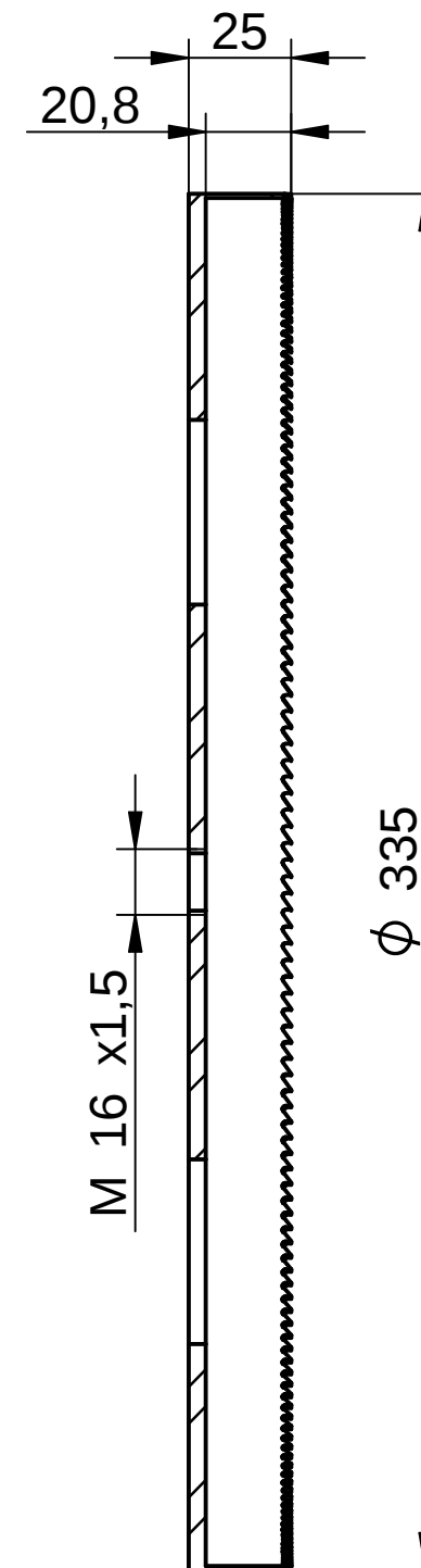
Schnitt A-A
