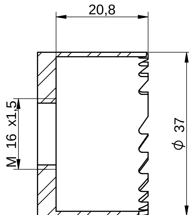
Schnitt A-A
