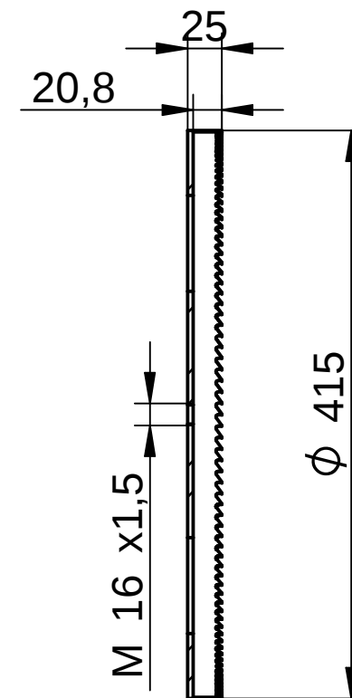
Schnitt A-A
