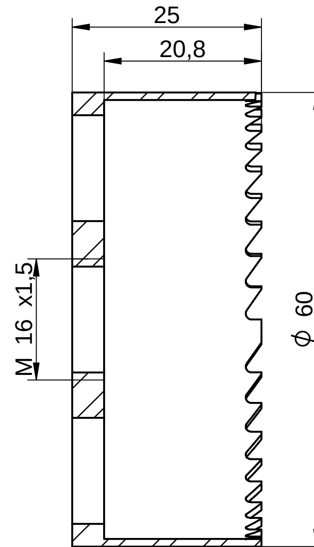
Schnitt A-A
