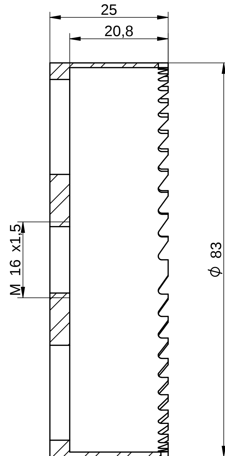
Schnitt A-A
