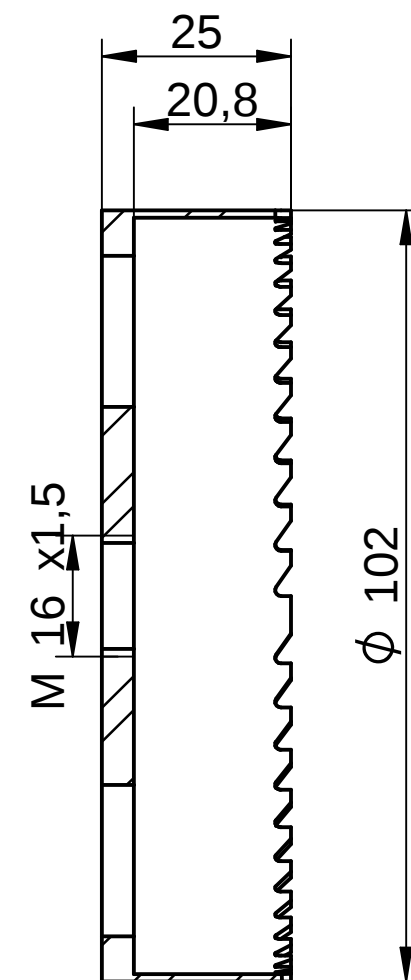
Schnitt A-A
