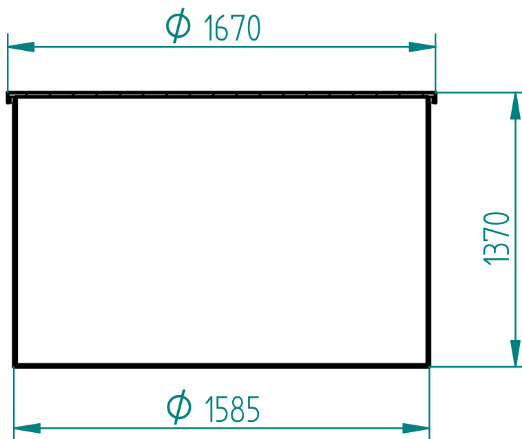
SCHNITT A-A
