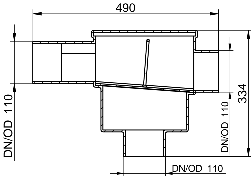
Schnitt A-A
