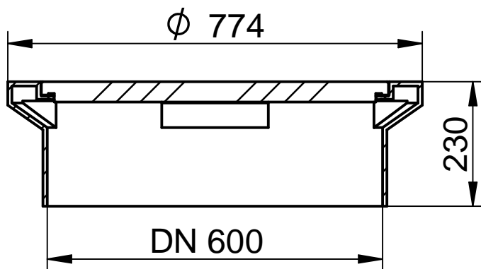
Schnitt A-A
